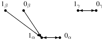
Diagram (d). \text{Cay}(S, \{1_\gamma\})
