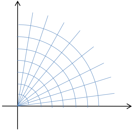
Polar coordinates
